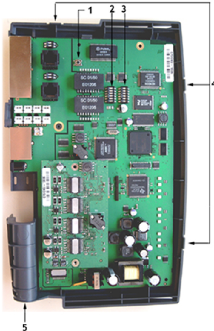
Figure 4-3 : e.Compact carte mère
